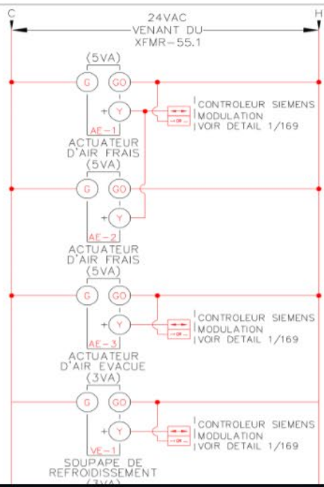
169 SYSTEME VA-02, VH-04A ET VH-04B SALLE GAZ MEDICAUX FD-SS-001
